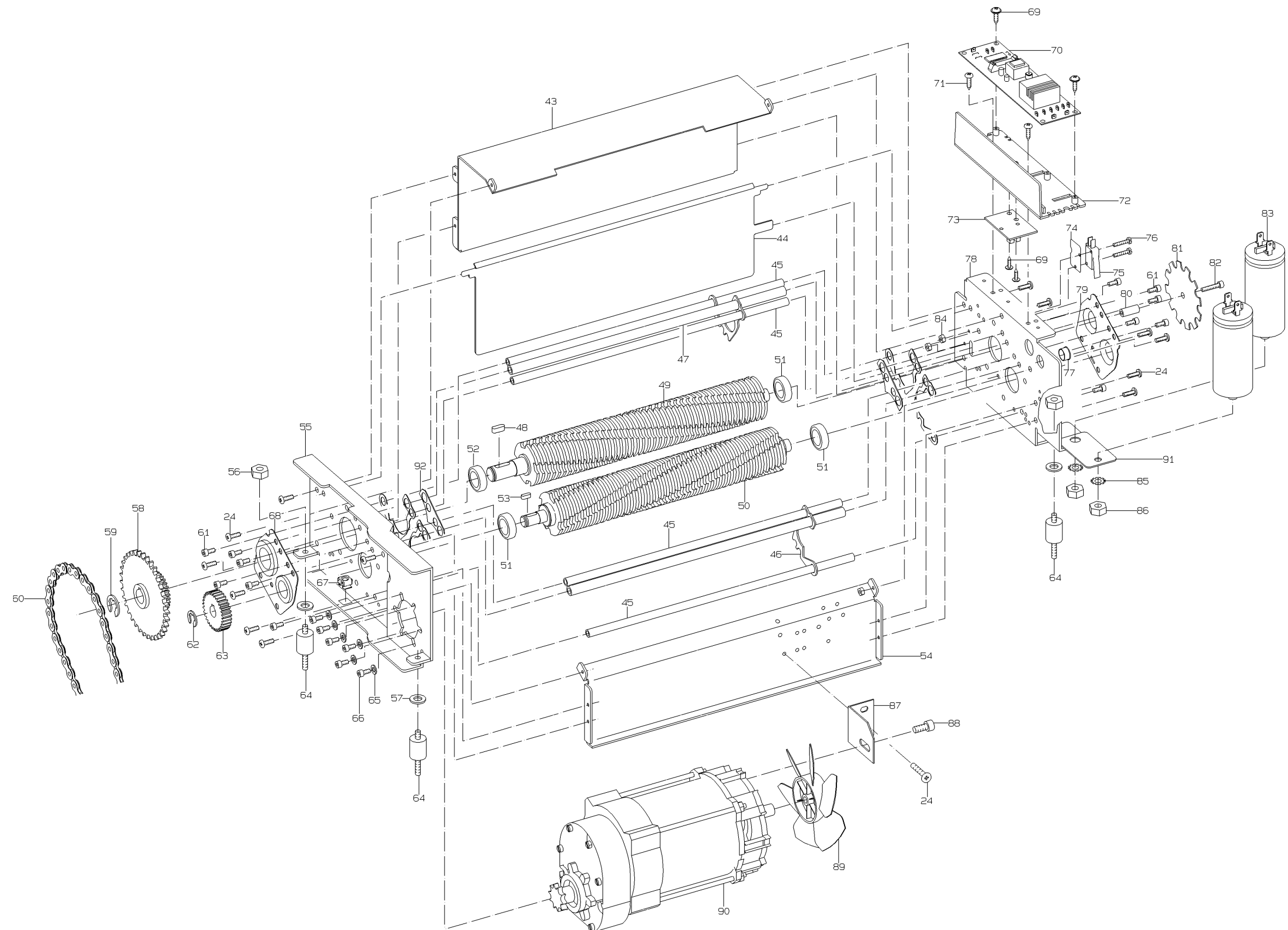
Abbildung 2 Aktenvernichter 33130 Illustration 2 Document shredder 33130 Illustration 2 Destructeur de documents 33130
