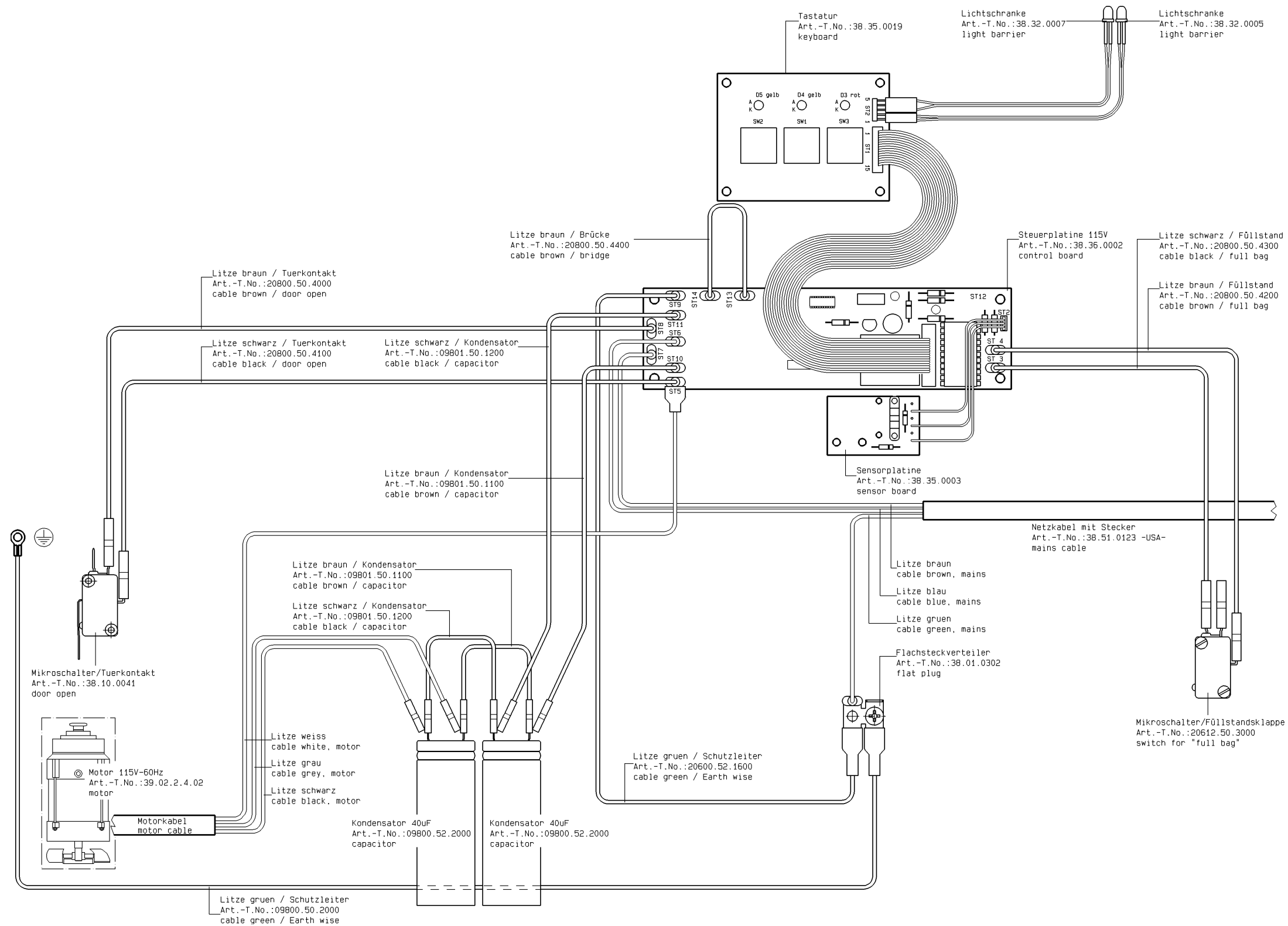
Abbildung 3 Schaltplan 33130 Illustration 3 Circuit diagram 33130 Illustration 3 Schéma électrique 33130
