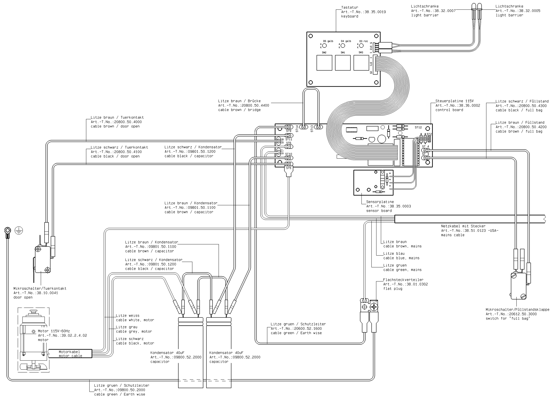
Abbildung 3 Schaltplan 33106 Illustration 3 Circuit diagram 33106 Illustration 3 Schéma électrique 33106
