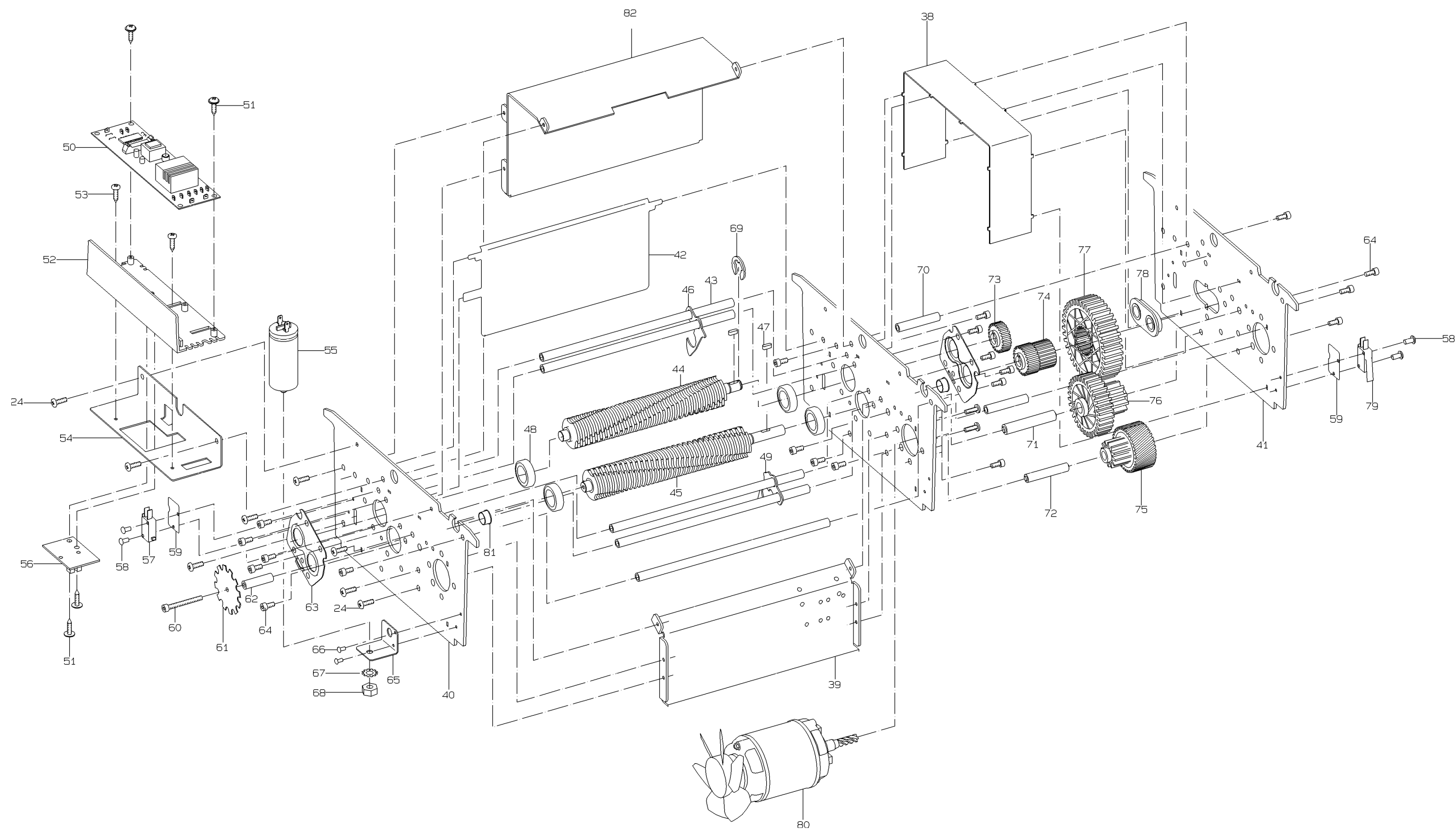
Abbildung 2 Aktenvernichter 32414 Illustration 2 Document shredder 32414 Illustration 2 Destructeur de documents 32414
