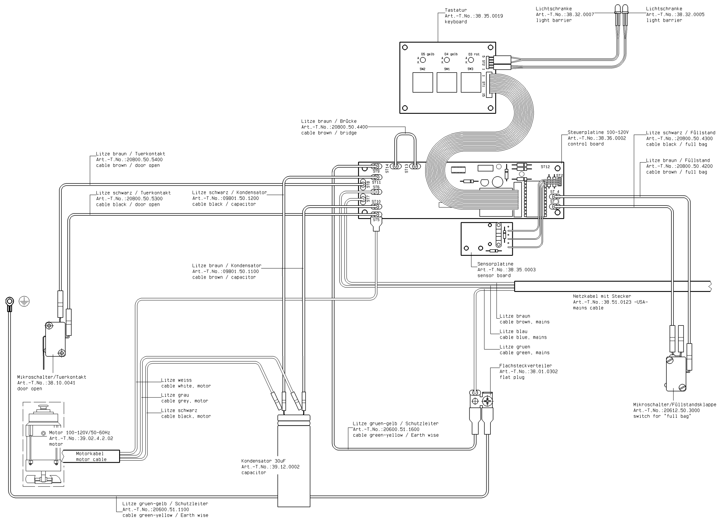
Abbildung 3 Schaltplan 32404 Illustration 3 Circuit diagram 32404 Illustration 3 Schéma électrique 32404
