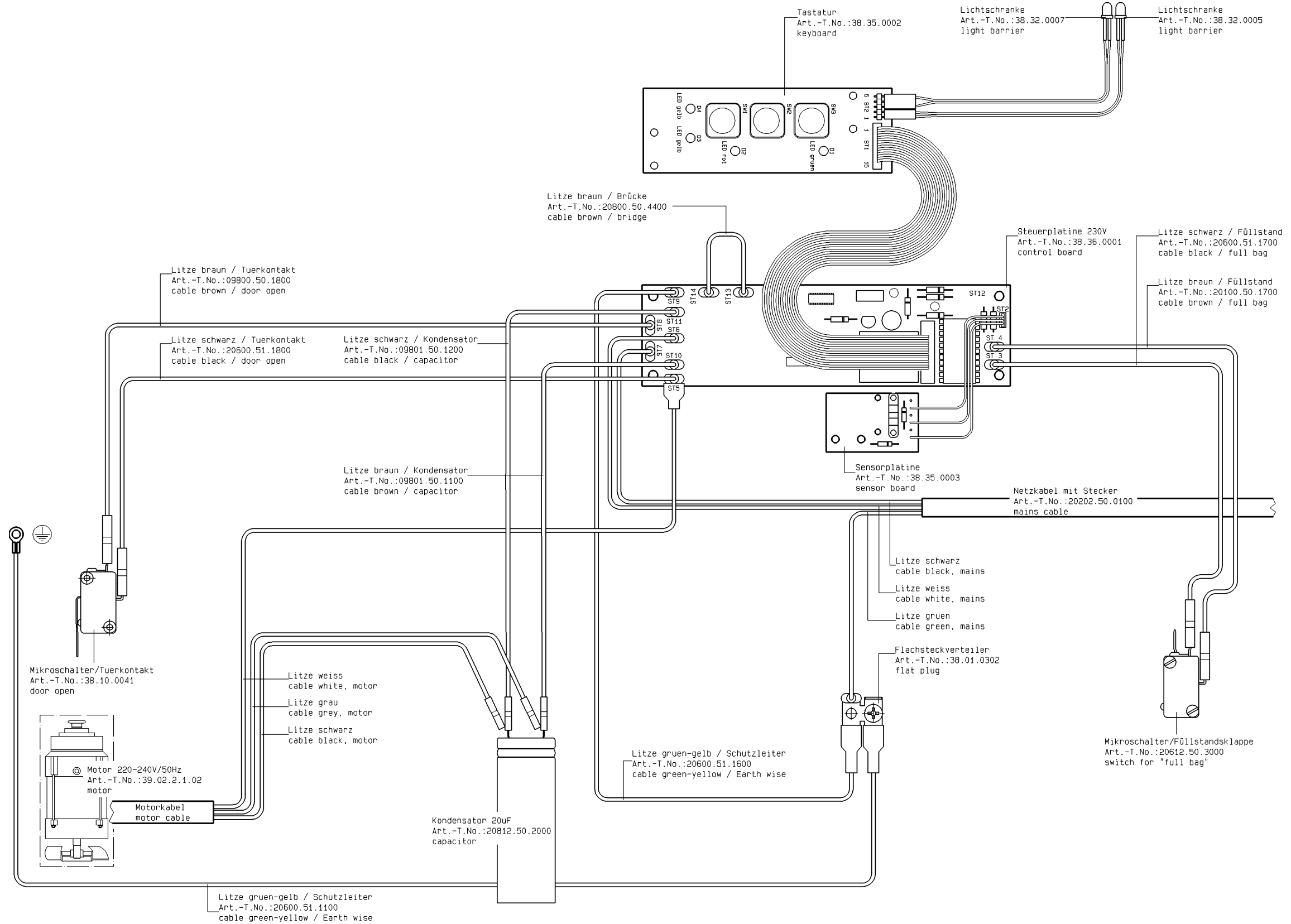
Abbildung 3 Schaltplan 20602 ME Illustration 3 Circuit diagram 20602 ME Illustration 3 Schéma électrique 20602 ME
