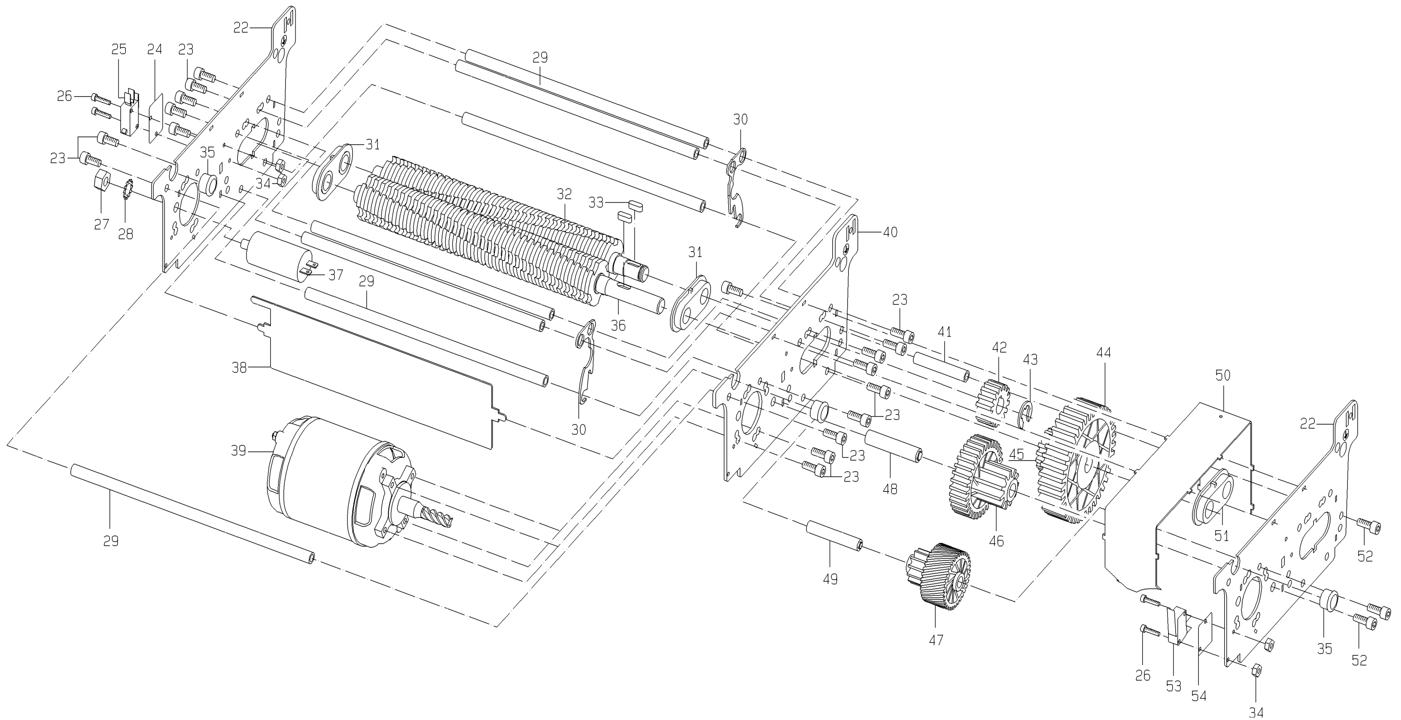
Abbildung 2 Aktenvernichter 20314 ELC Illustration 2 Document shredder 20314 ELC Illustration 2 Destructeur de documents 20314 ELC
