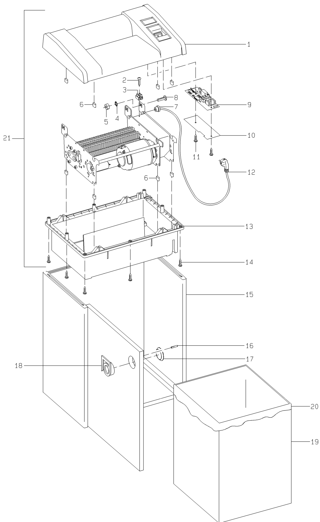
Abbildung 1 Aktensvernichter 20304 ES Illustration 1 Document shredder 20304 ES Illustration 1 Destructeur de documents 20304 ES
