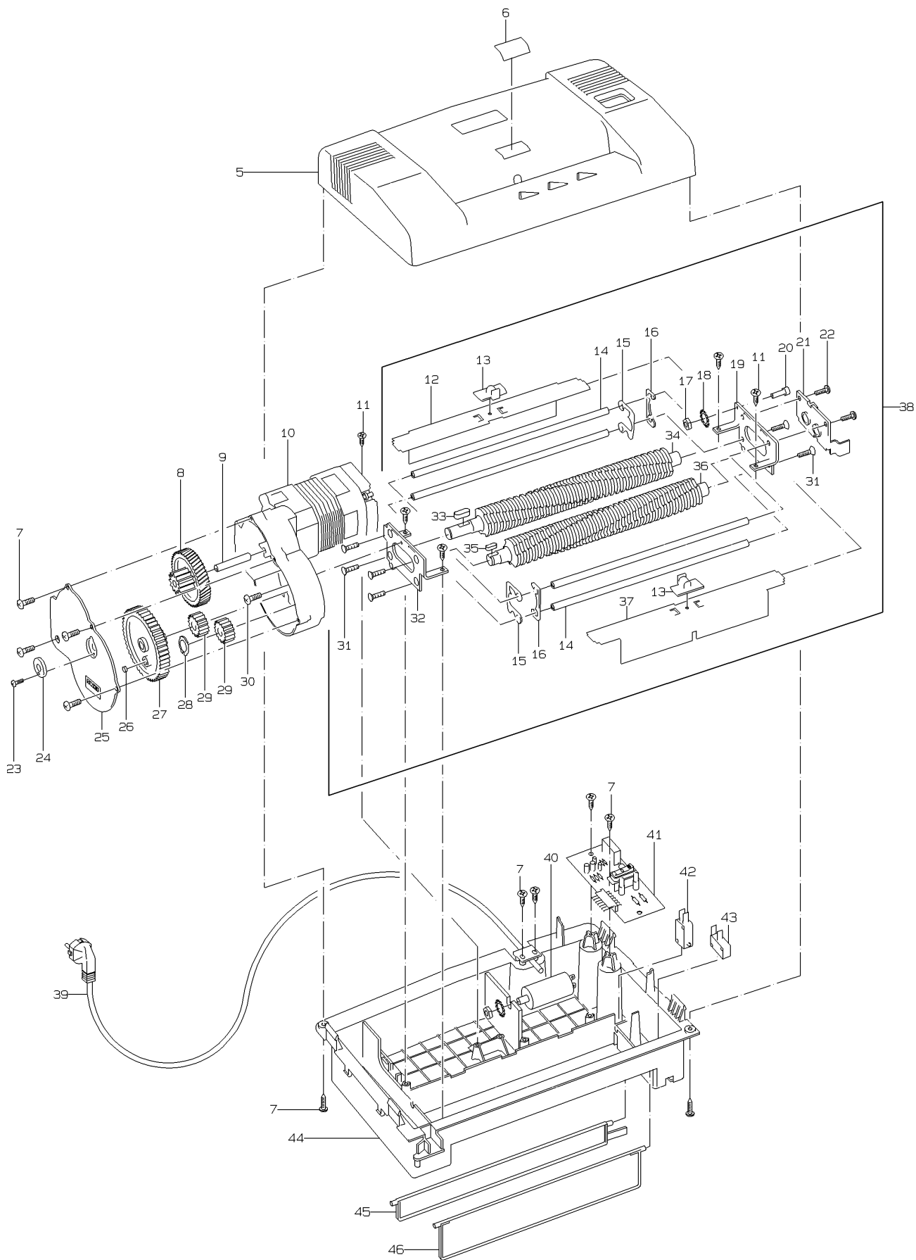
Abbildung 2 Aktensvernichter 20120 LEC Illustration 2 Document shredder 20120 LEC Illustration 2 Destructeur de documents 20120 LEC
