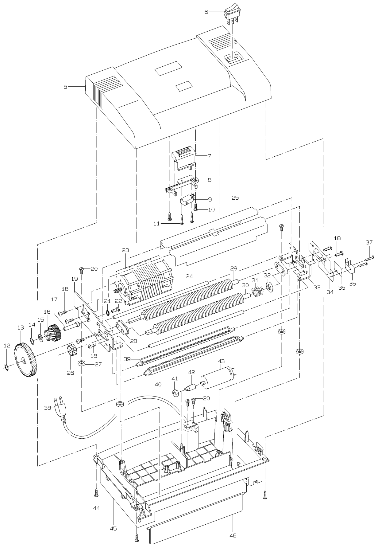
Abbildung 2 Aktenvernichter 20100 PS Illustration 2 Document shredder 20100 PS Illustration 2 Destructeur de documents 20100 PS
