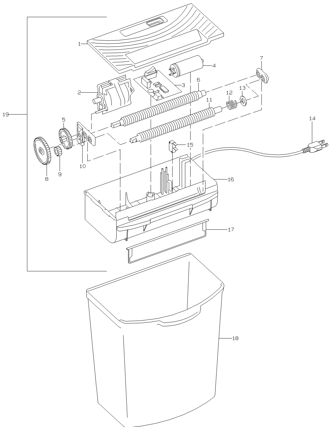
Abbildung 1 Aktensvernichter 20050 eco Illustration 1 Document shredder 20050 eco Illustration 1 Destructeur de documents 20050 eco
