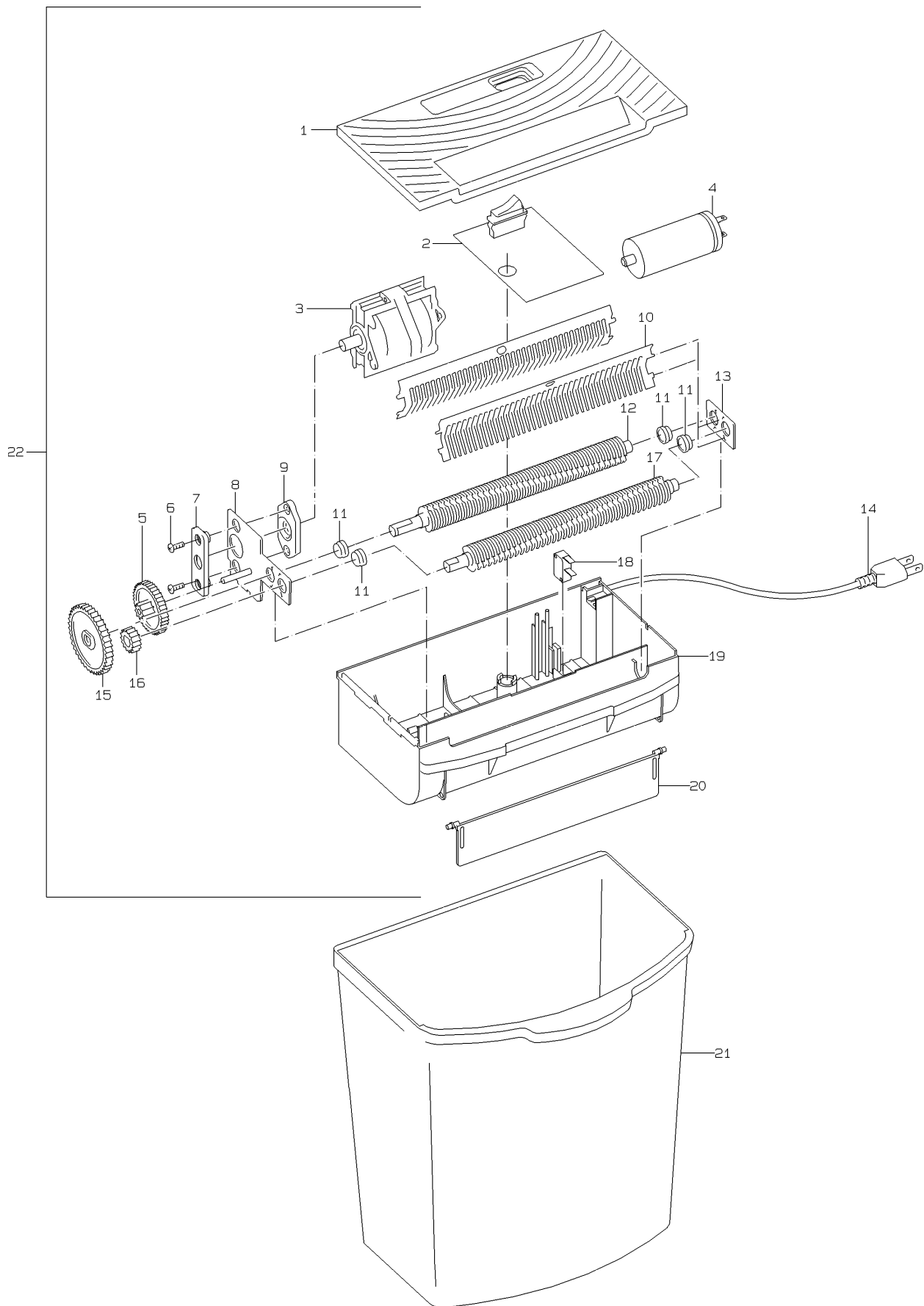
Abbildung 1 Aktenvernichter 20032 ecoC Illustration 1 Document shredder 20032 ecoC Illustration 1 Destructeur de documents 20032 ecoC
