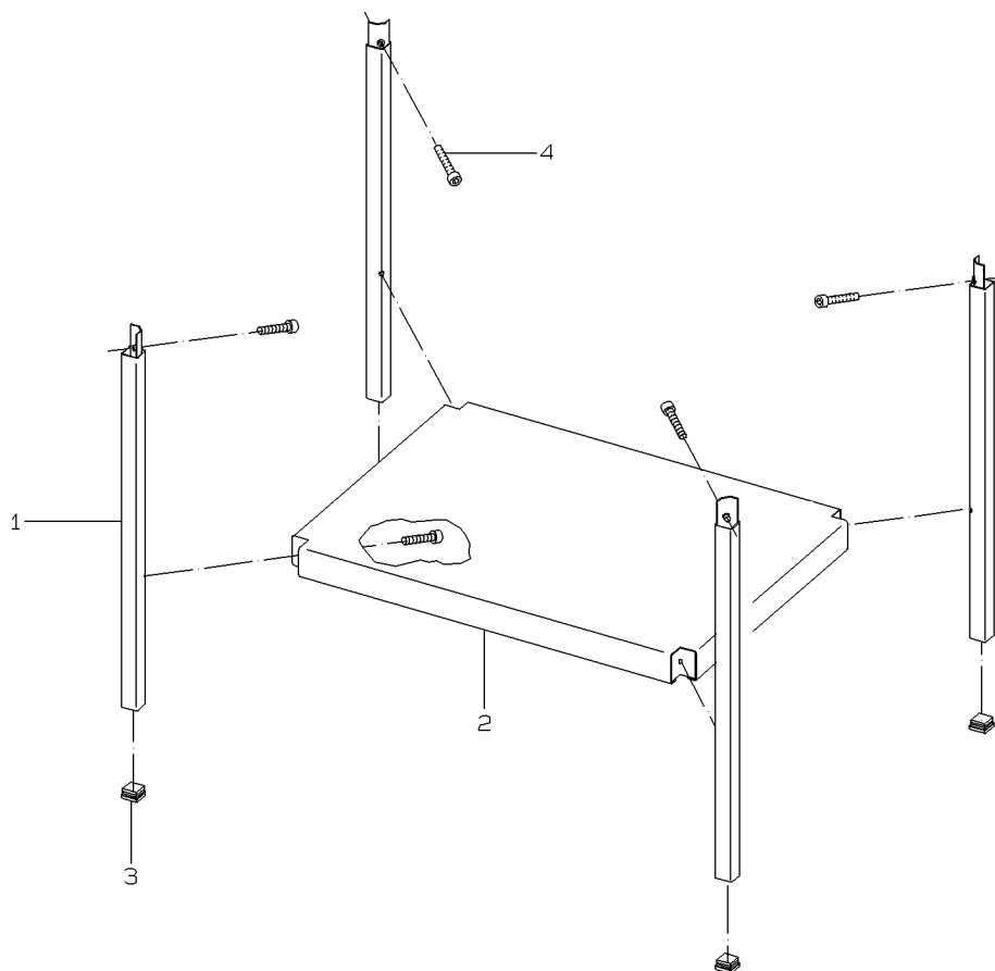
Abbildung 2 Untergestell 619
